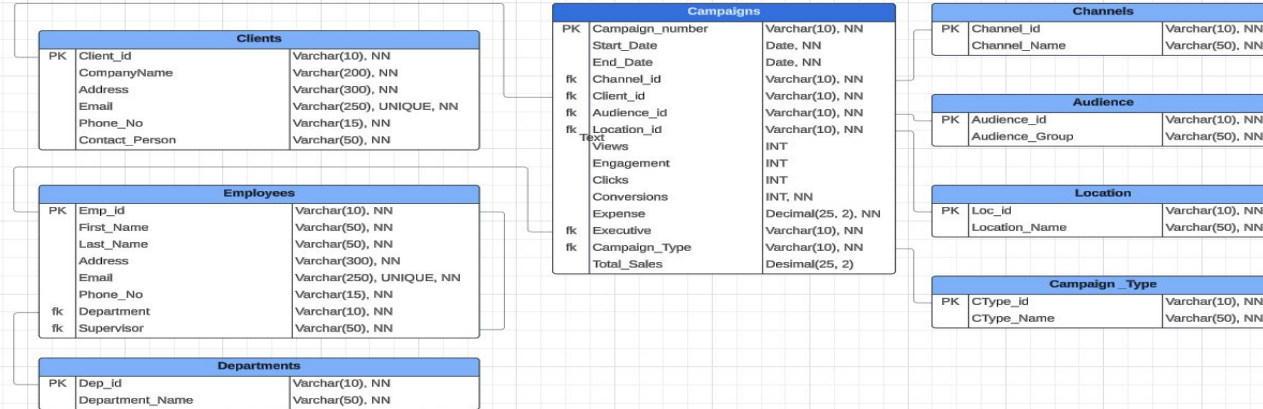
MarketFlash ER Diagram
